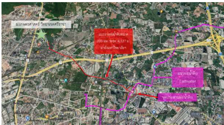
ภาพที่ 2 แสดงแนวเส้นทางวางท่อน้ำดิบขนาด 200 มม. จากสี่แยกศรีสุพรรณถึงมหาวิทยาลัยเกษตรศาสตร์ วิทยาเขตศรีราชา
